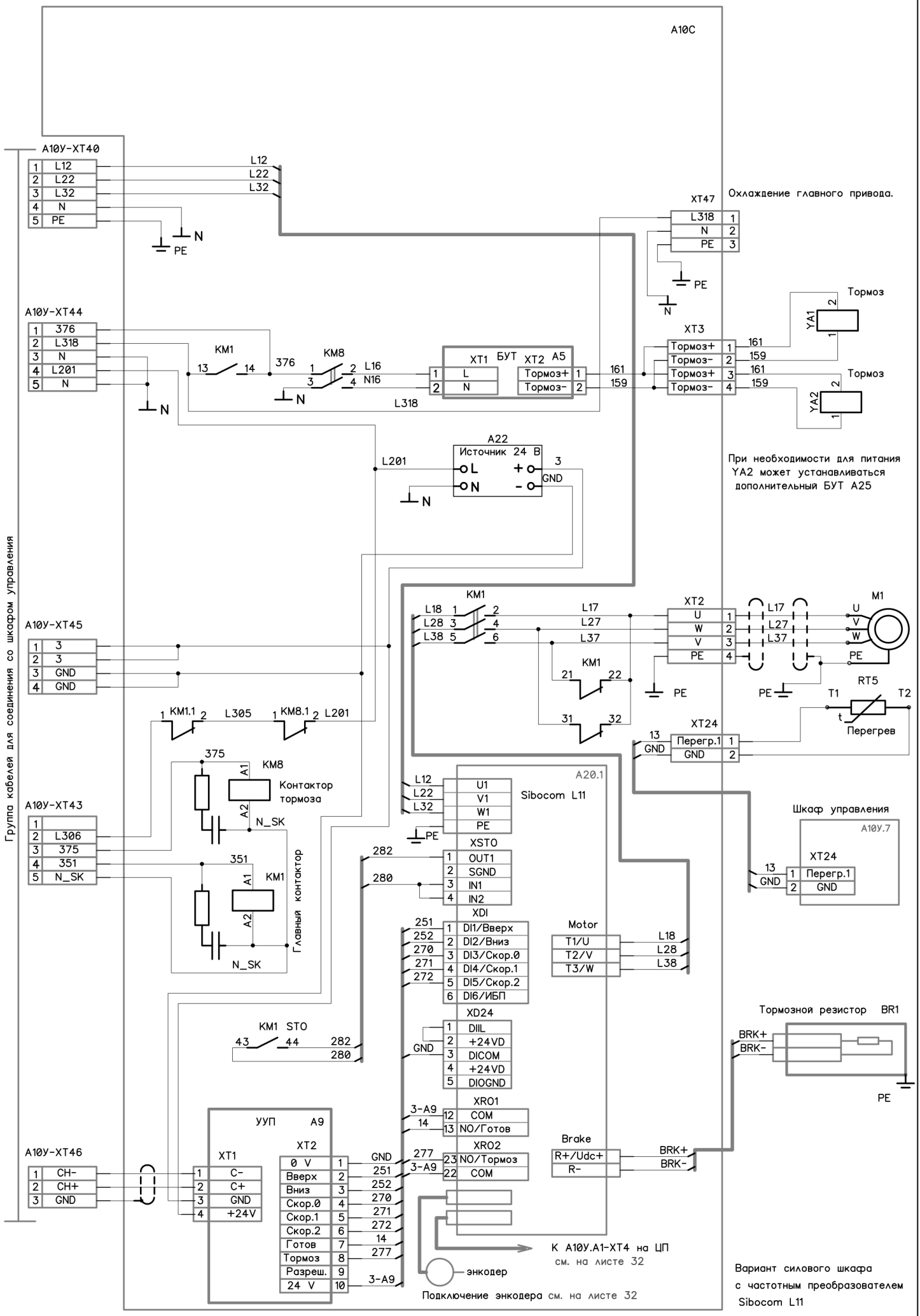
Вариант схемы без автоматической эвакуации.
